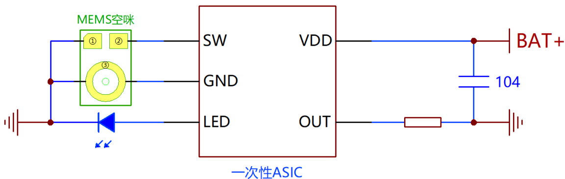
图示 4. MEMS 空咪与一次性 ASIC 配合
