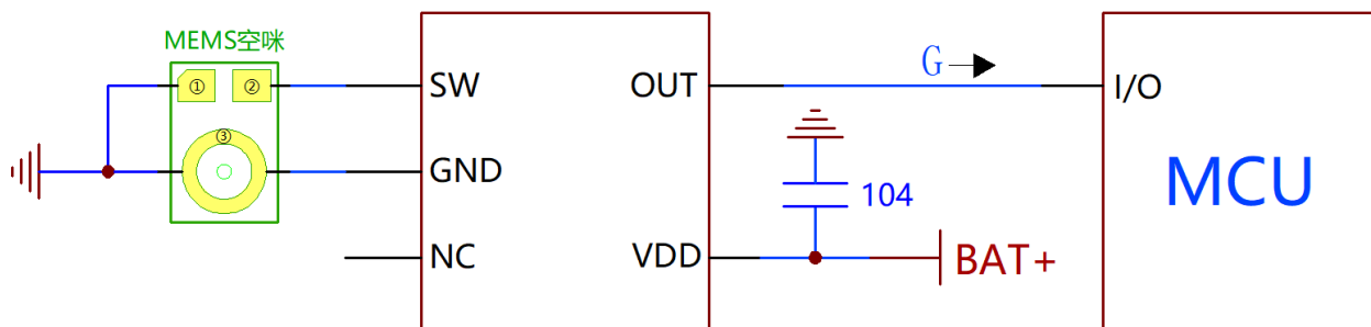
图示 3. MEMS 空咪与换弹 ASIC 配合
