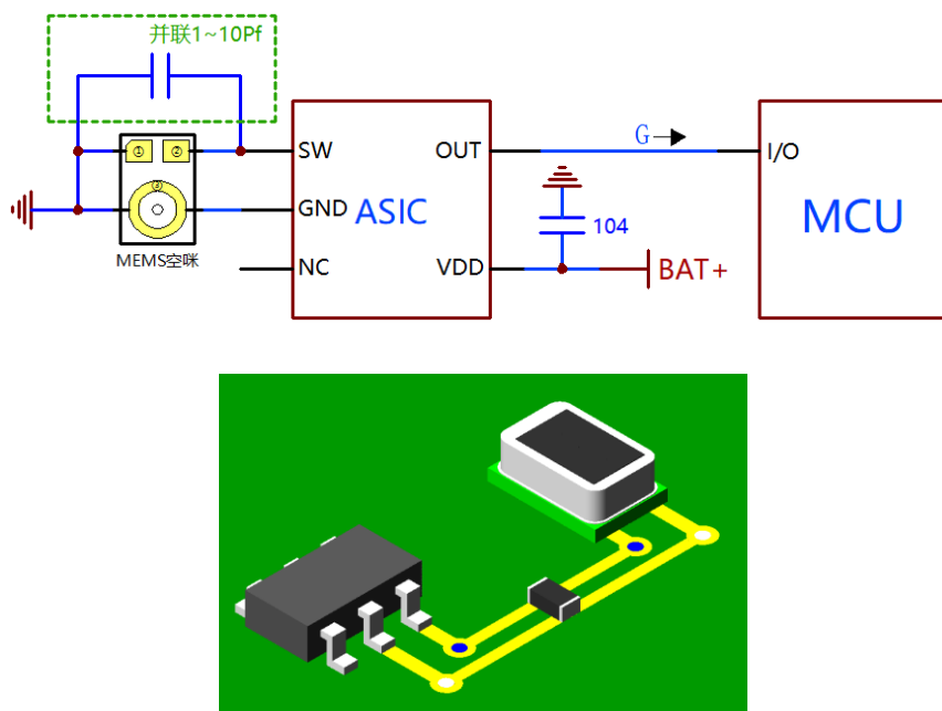
图示 6. 应用电路示意图
