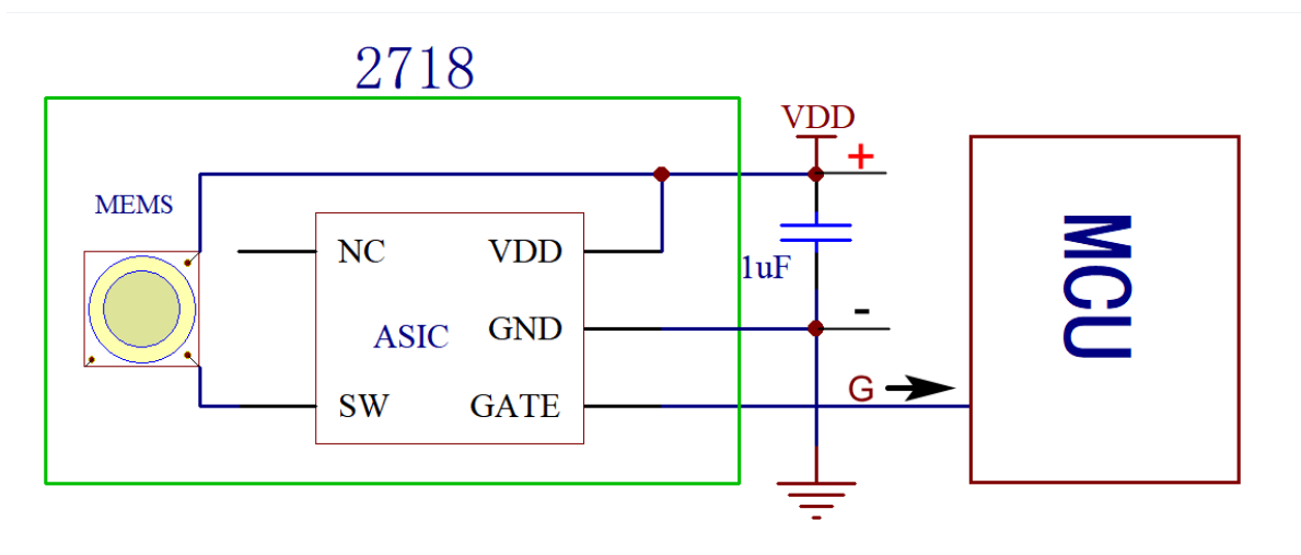
图示 3. 应用原理图
