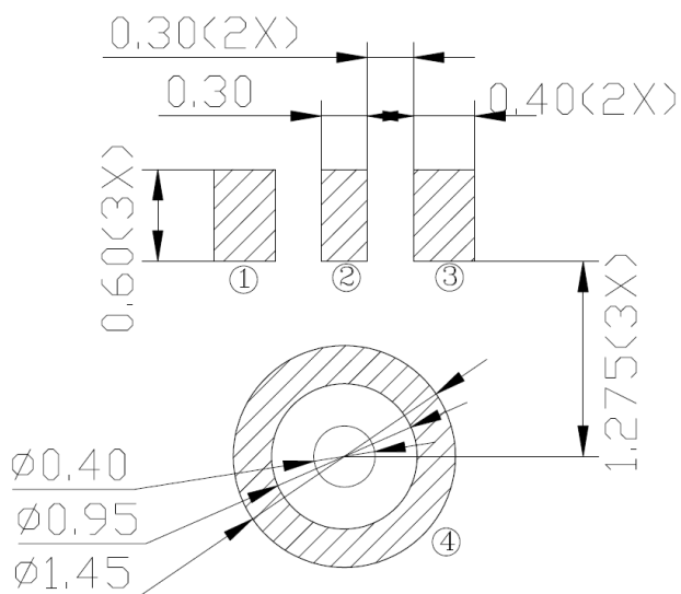
图示 2. 推荐客户端 PCB 开窗图纸
