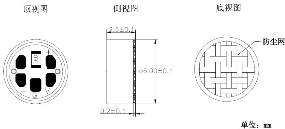
图示 1. 外形尺寸图
