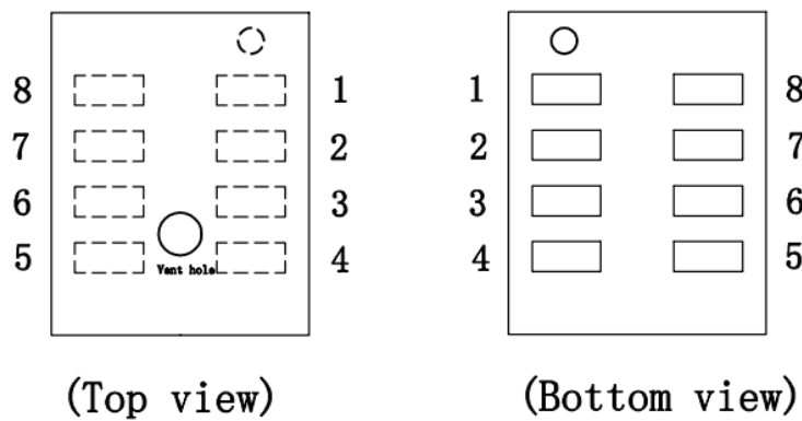
图6: 引脚配置图
