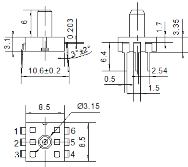
图6: 引脚配置图
